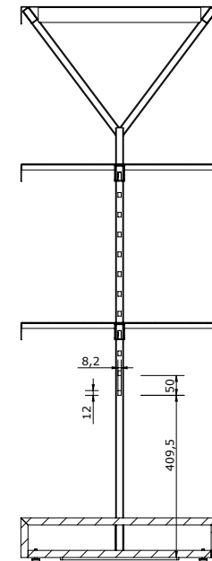
Section A-A Scale 1 : 10
